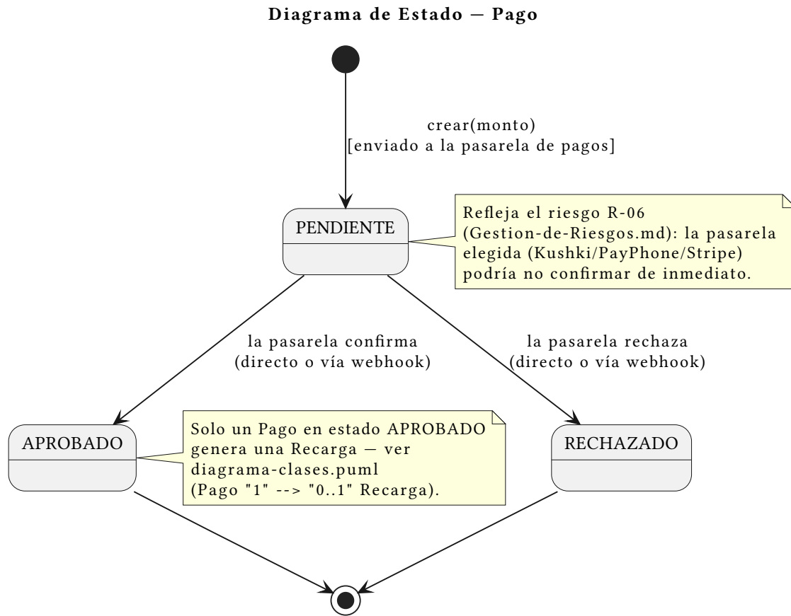
Figure 12: Estado: Pago
